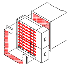
Fig. 3 —sch—ma d'installation de deux appareils groupés dans une conduite.
