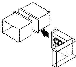
Fig. 1 —sch—ma d'installation pour appareil x brides.
