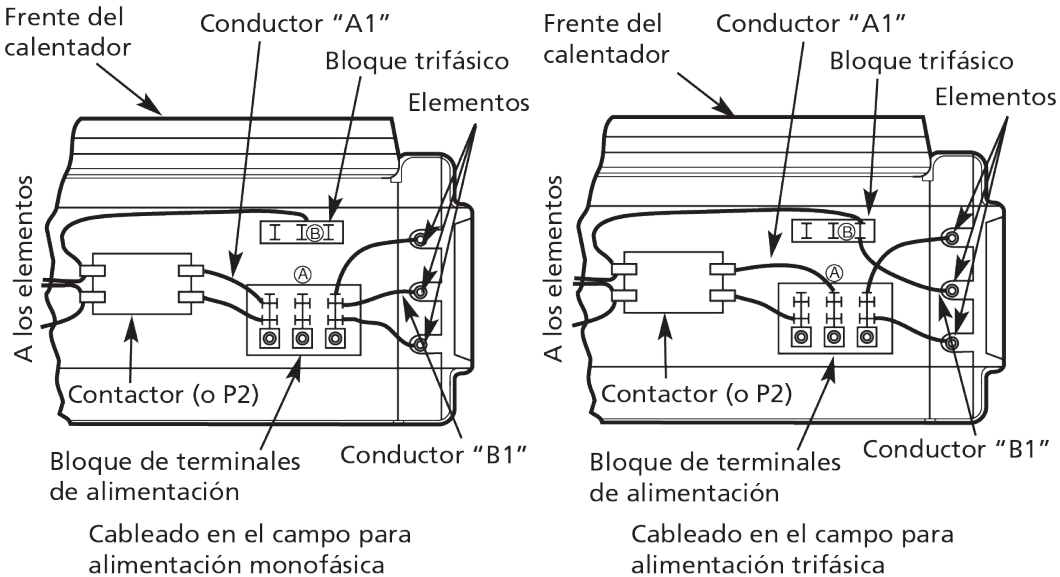
Figura 3a. Conexiones de cables para alimentación monofásica y trifásica (MUH0321, MUH0521, MUH0581)
