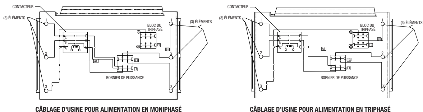
Figure 3b. Raccordements d'alimentation pour du secteur monophasé et triphasé (MUH072, MUH078, MUH102, MUH108)
