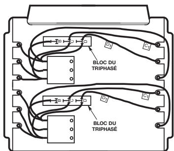
CÂBLAGE D'USINE POUR ALIMENTATION EN MONOPHASE
