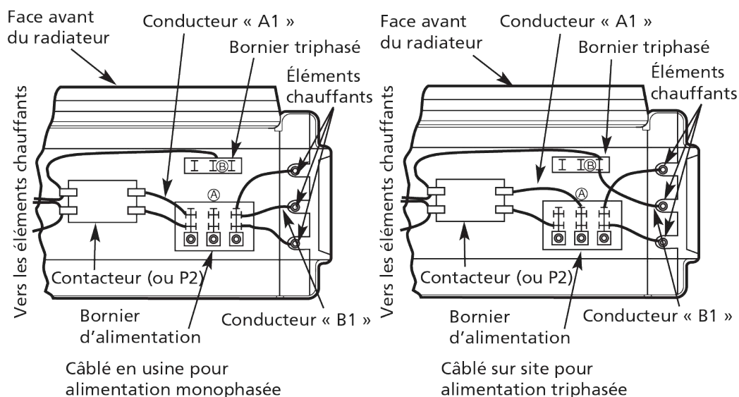
Figure 3a. Raccordements d'alimentation pour du secteur monophasé et triphasé (MUH0321, MUH0521, MUH0581)
