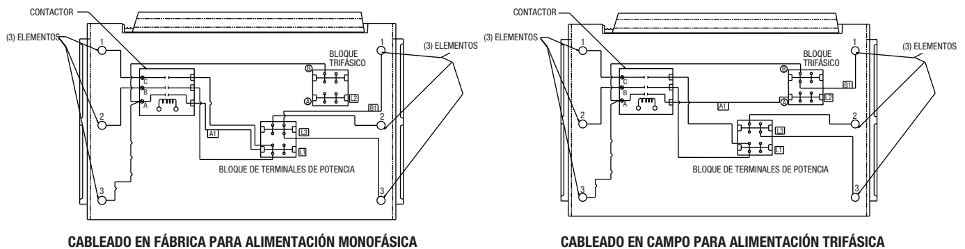
Figura 3b. Conexiones de cableado para alimentación monofásica y trifásica (MUH072, MUH078, MUH102, MUH108)
