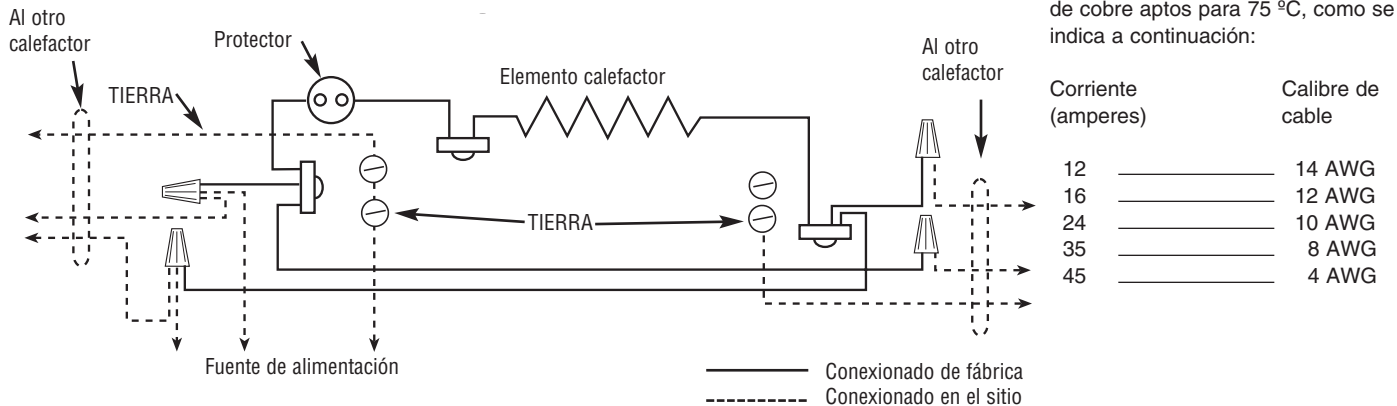
Fig. 2 Diagrama de conexonado
