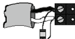
Figure 9: Détail de la résistance de terminaison
